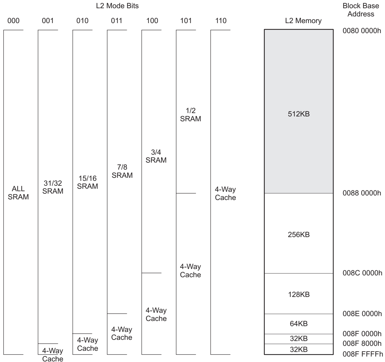
图 6-4. L2 Memory Configurations
