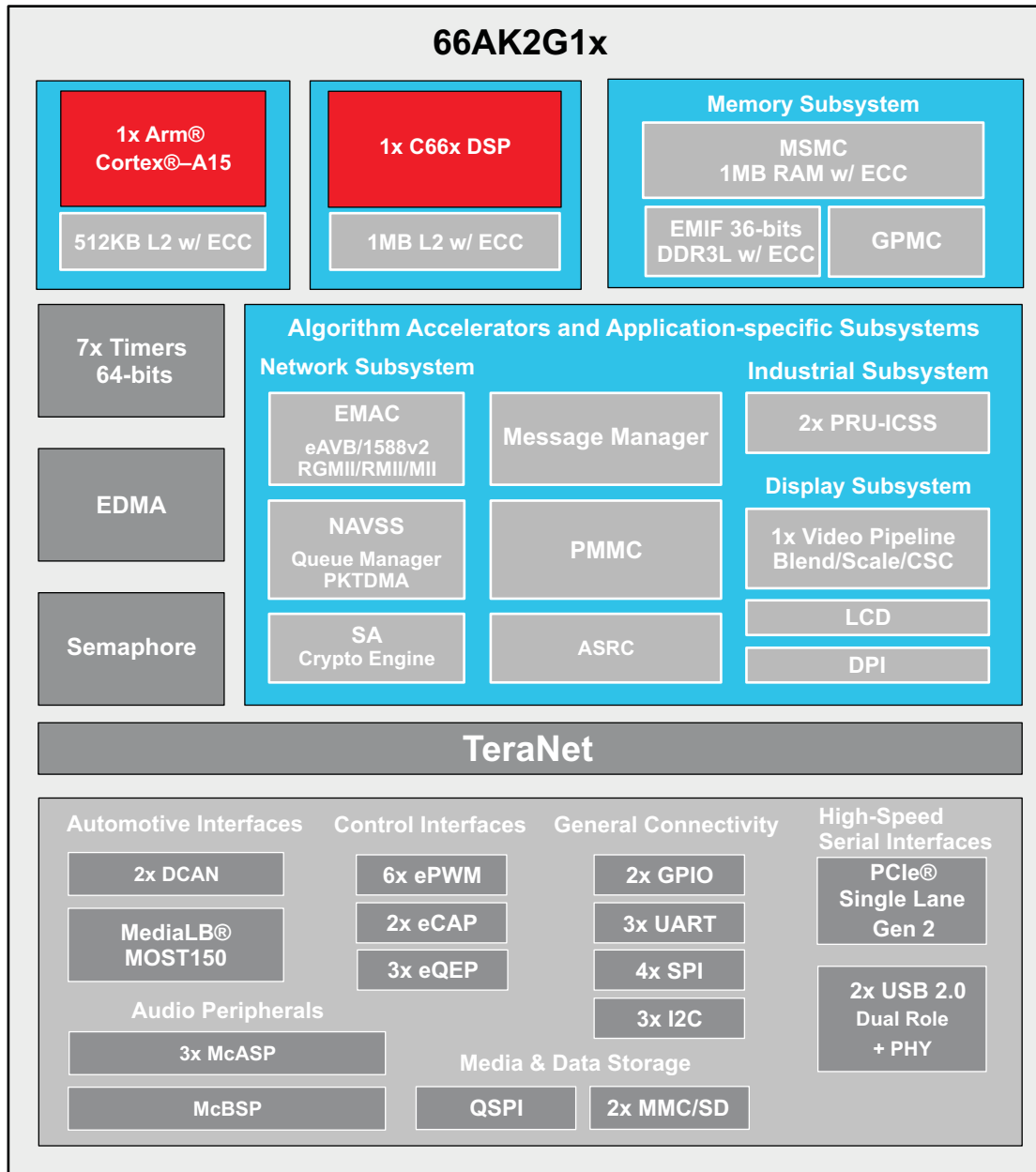
图 1-1. 功能方框图
