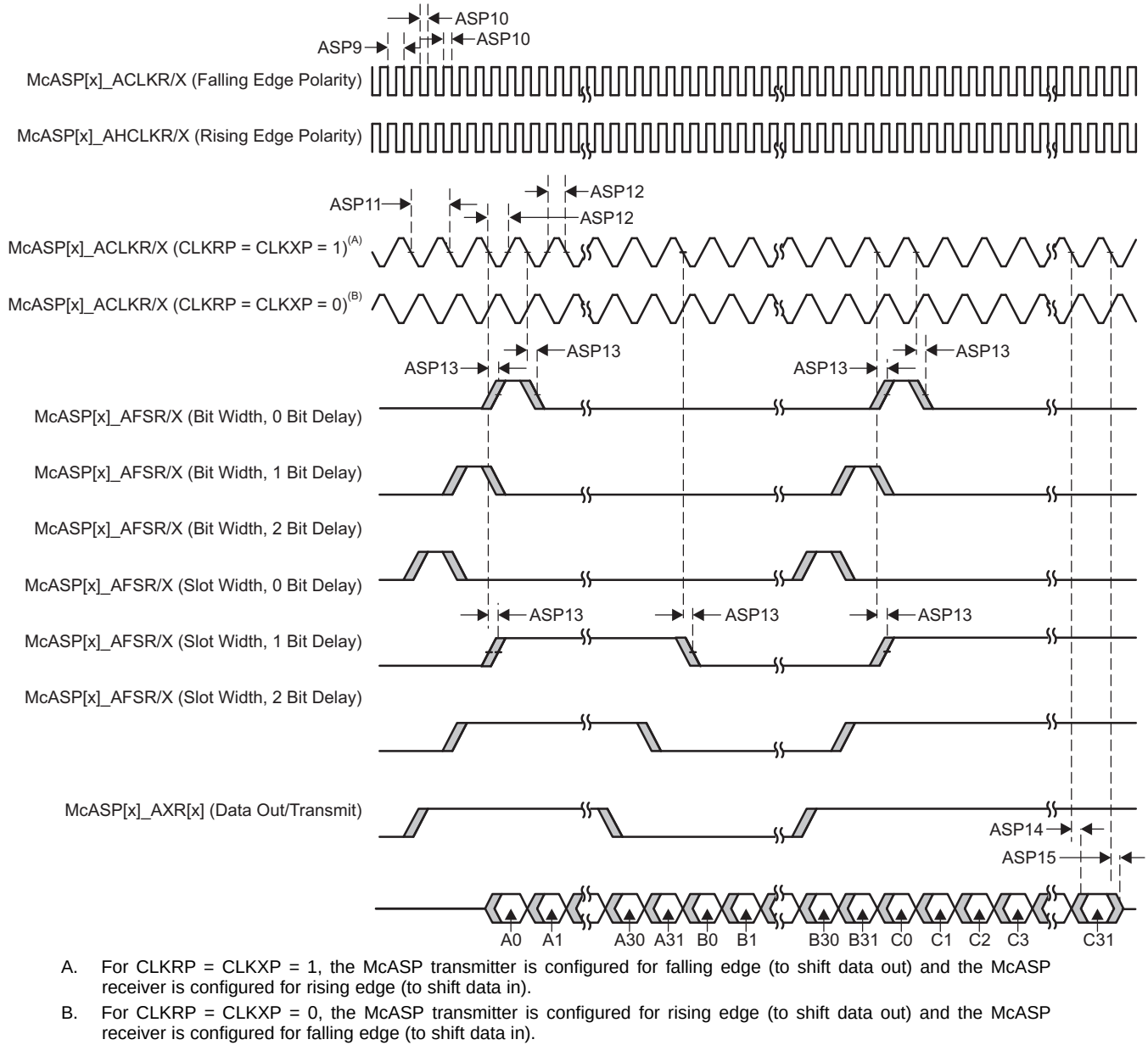
图 5-50. McASP Output Timing
