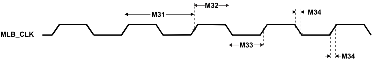
图 5-53. MLB_CLK Timing
