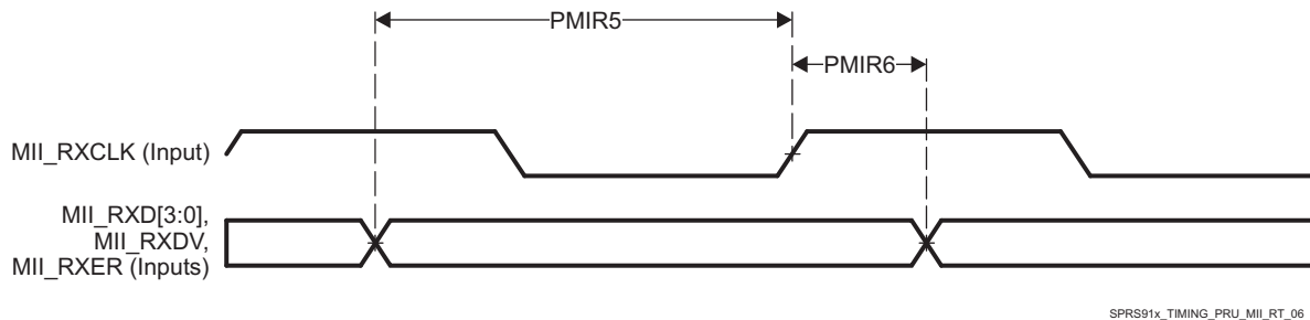
图 5-76. PRU-ICSS MII_RXD[3:0], MII_RXDV, and MII_RXER Timing
