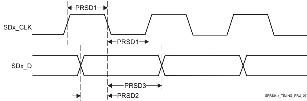
图 5-79. PRU-ICSS PRU SD_CLK Falling Active Edge
